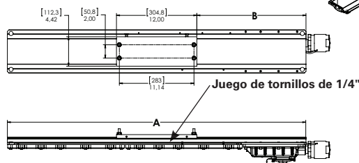
Figura 3. ZP1057MTK Instalación del montaje posterior
